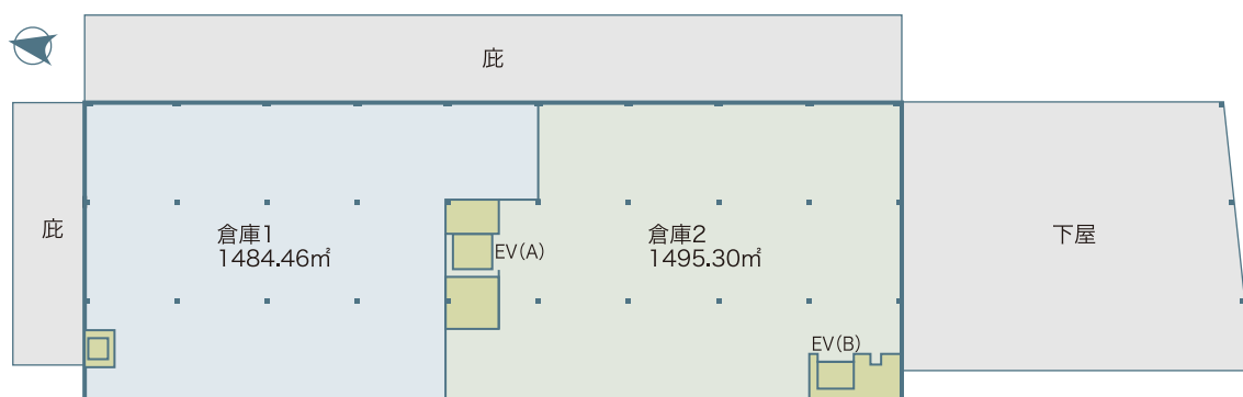
2階 平面図
