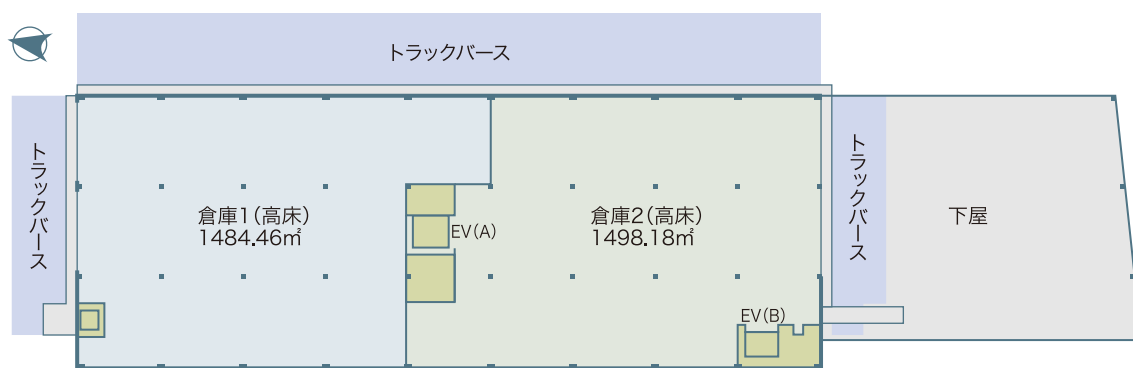
1階 平面図
