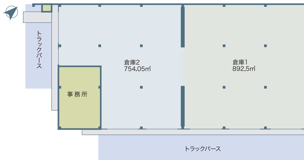
1階 平面図
