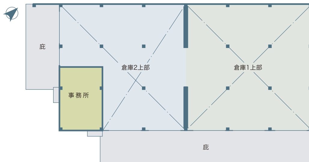
2階 平面図
