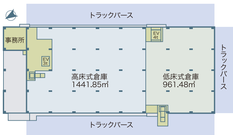
1階 平面図
